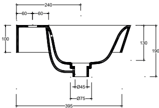
Sezione A-A Section A-A
